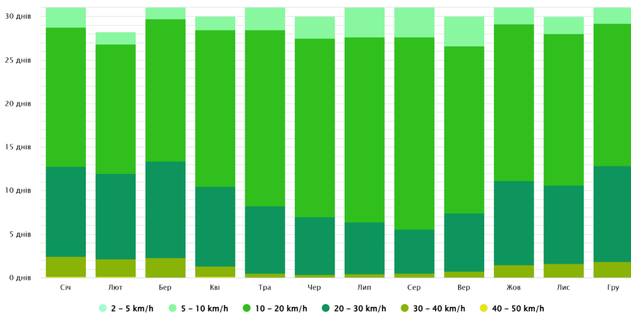
Рис. 6. Швидкість вітру
