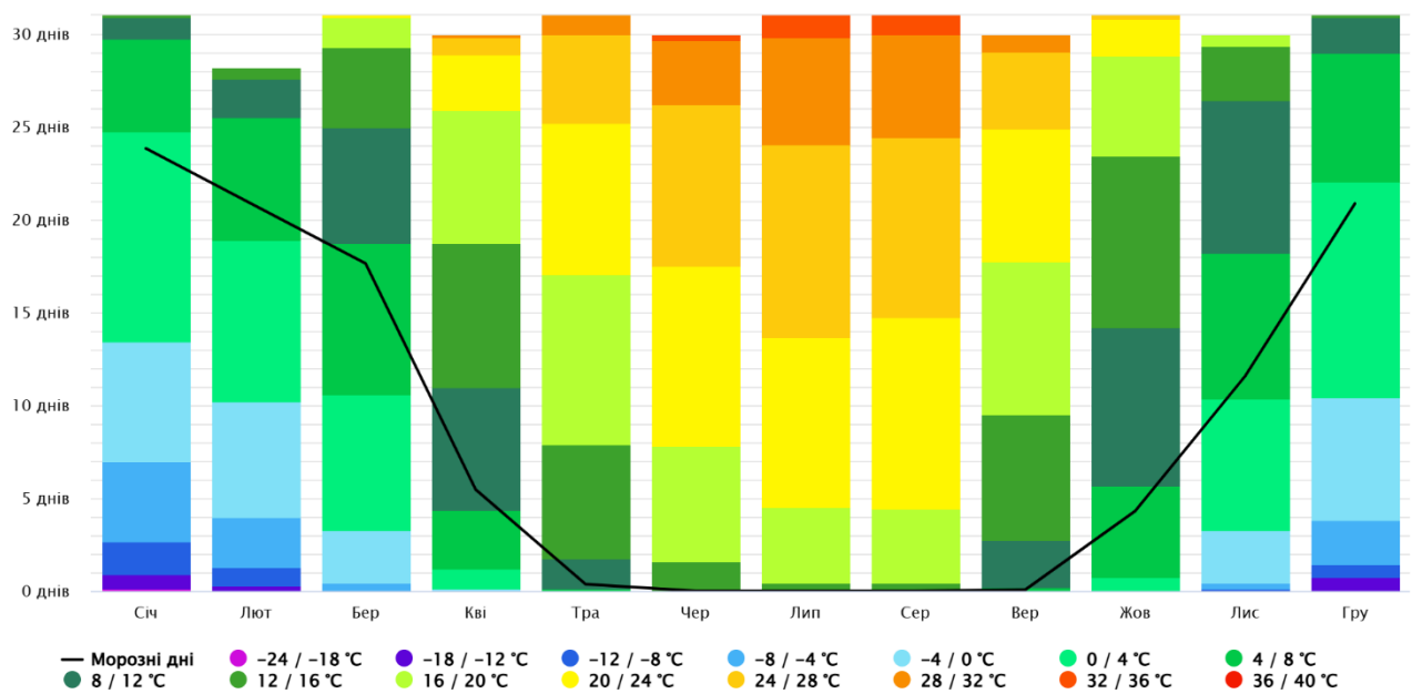
Рис. 4. Максимальні температури
