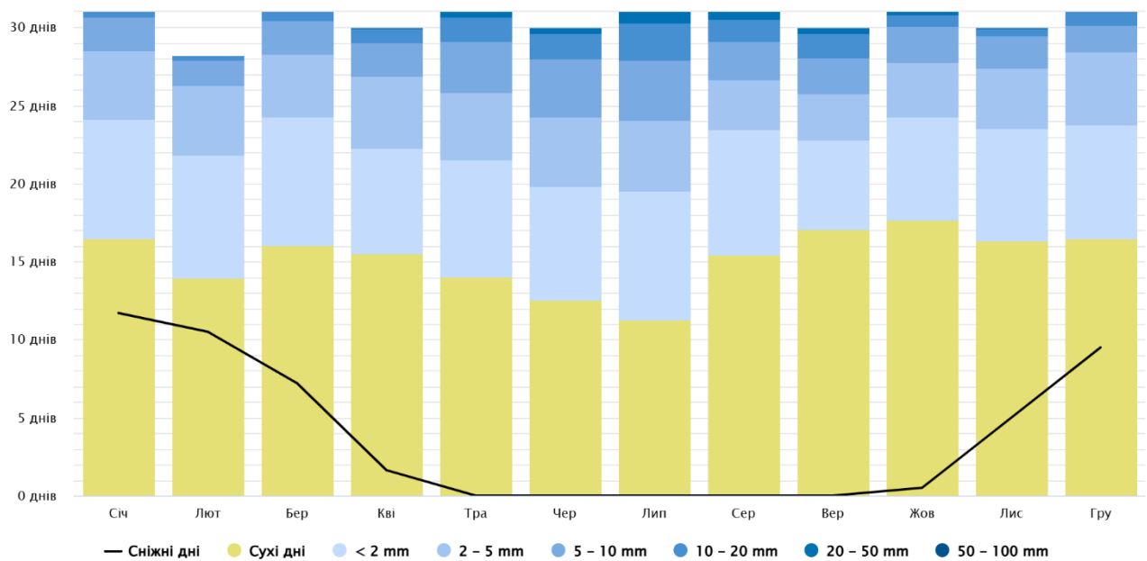
Рис. 5. Кількість опадів
