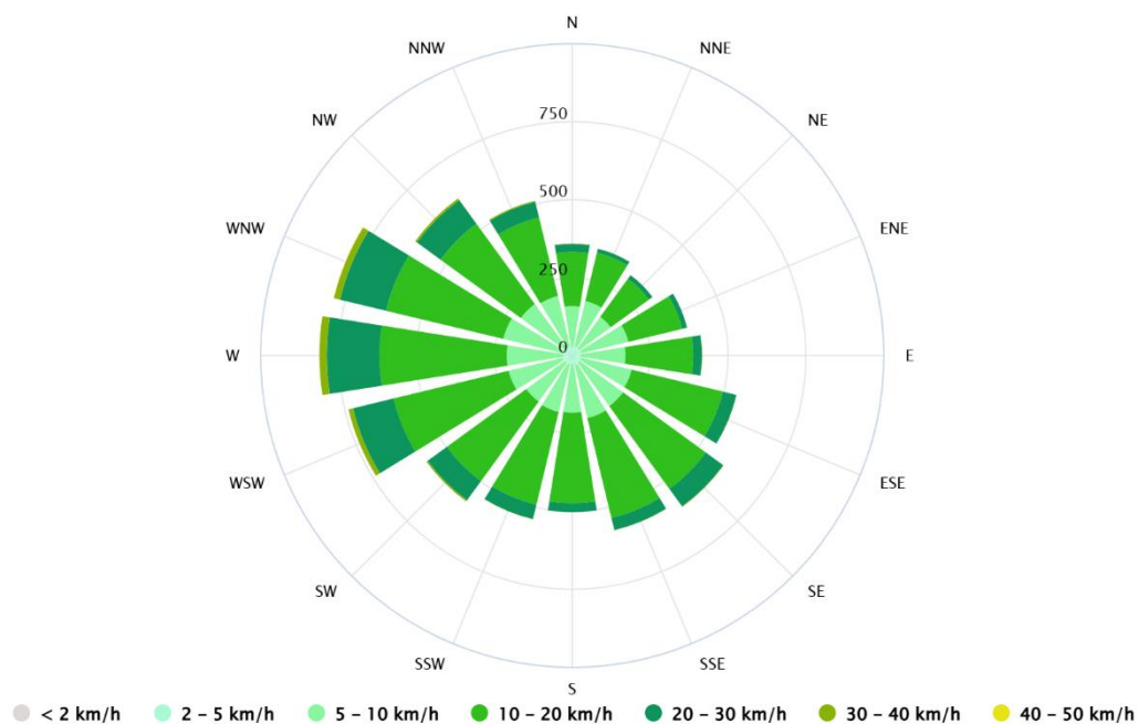
Рис. 7. Роза вітрів
